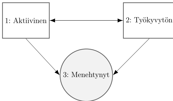
Kuva 5.3: Kolmitilainen markovilainen prosessi. Tilat kuvaavat vakuutetun työkykyisyyttä. Aktiivinen vakuutettu voi joutua työkyvyttömäksi tai menehtyä. Työkyvyttö voi palata aktiiviseksi tai menehtyä. Menehtynyt ei luonnollisesti voi enää herätä henkiin.
