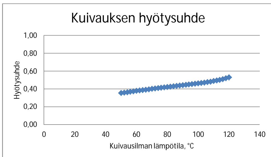
Kuva 19. Kuivausilman lämpötilan vaikutus kuivauksen hyötysuhteeseen.
