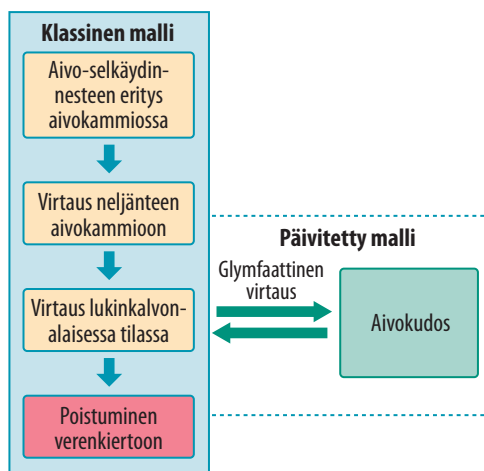
KUVA 2. Aivo-selkäydinnesteen kierron klassinen malli ja glymfaattisen kierron huomioiva päivitetty malli. Aivo-selkäydinneste erittyy sivukammioissa ja kolmannessa aivokammiossa, joista se virtaa neljännen aivokammion kautta lukinkalvonalaisen tilaan. Osa aivo-selkäydinnesteestä päätyy glymfaattisen virtauksen mukana puhdistamaan aivokudosta. Aivokudoksen kautta kiertävän nesteen tilavuusosuus vaihtelee fysiologisen tilan mukaan. Aivokudoksesta neste laskee jälleen lukinkalvonalaisen aivo-selkäydinnestetilaa ja poistuu edelleen verenkiertoon.
