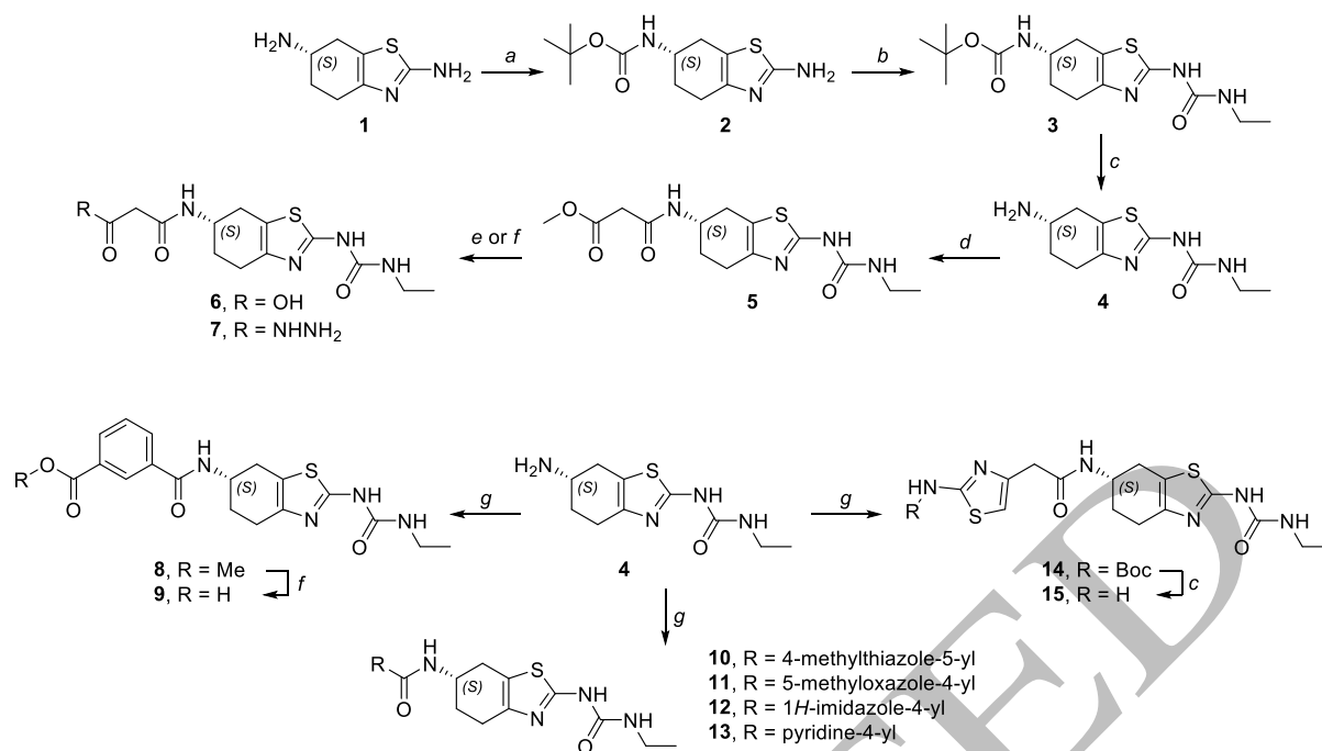
Scheme 1. Reagents and conditions. (a) Boc 2 O, THF, r.t., 18 h. (b) Ethyl isocyanate, CHCl 3 , r.t., 18 h. (c) Acetyl chloride, MeOH, 0 °C, 1 h, then r.t., 18 h. (d) Methyl malonyl chloride, Et 3 N, 1,4-dioxane, r.t., 18 h. (e) 6 : 1 M NaOH, MeOH/H 2 O, r.t., 24 h. (f) 7 : hydrazine hydrate, EtOH, 80 °C, 18 h. (g) Carboxylic acid, EDC, HOBt, NMM, DMF, r.t., 24 h.
