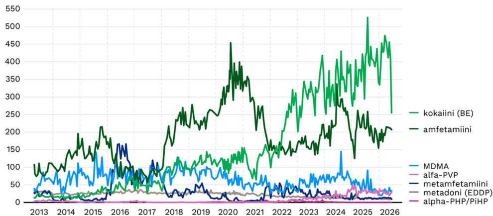
Kuvio 3. Huumejäämät Helsingin Viikinmäen jätevedenpuhdistamolla (noin 940 000 asukasta) ajanjaksolla 2013–2026 ilmoitettuna yksikössä milligrammaa (huumejäämä)/1000 henkilöä/päivä. Lähde: THL (2026b)
